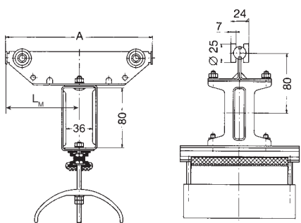
Ausführung mit Puffer
