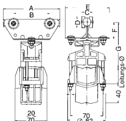
Ausführung mit Puffer
