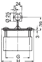
Ausführung mit Puffer
